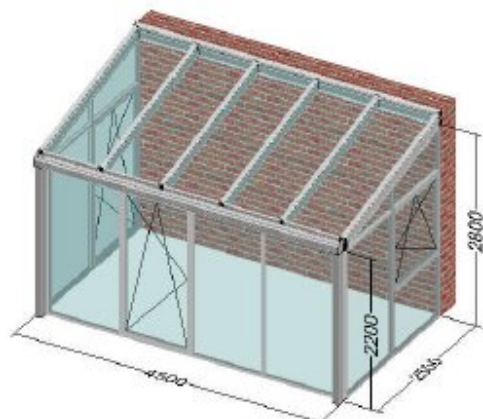
Vorderansicht Perspektive
